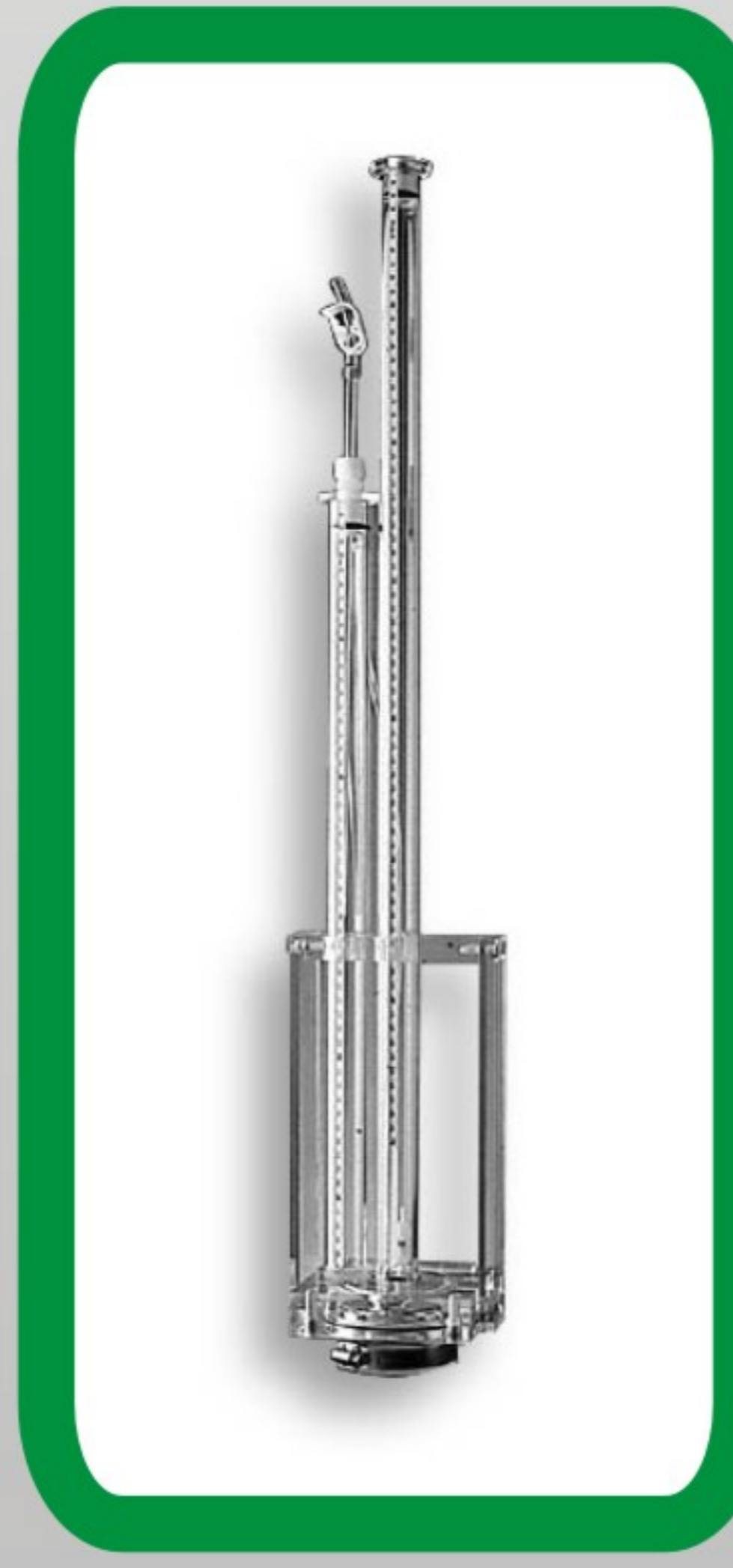
Wooding İnfiltrometre *Doymuş Toprakta Hidrolik İletkenlik Ölçümü
